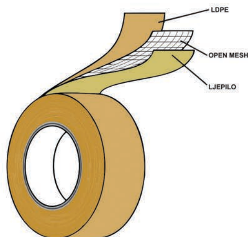
STANDARDNA KONSTRUKCIJA DUCT TRAKA
